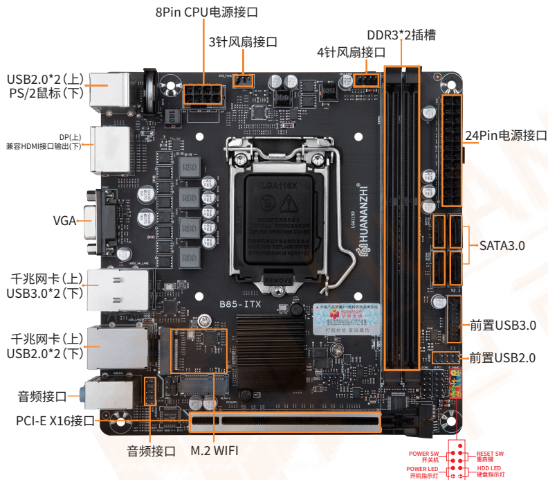
图1-1 B85-ITX 主板图解
