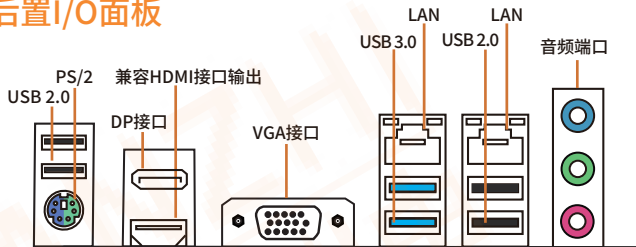
图1-2 整体后置I/O面板展示
